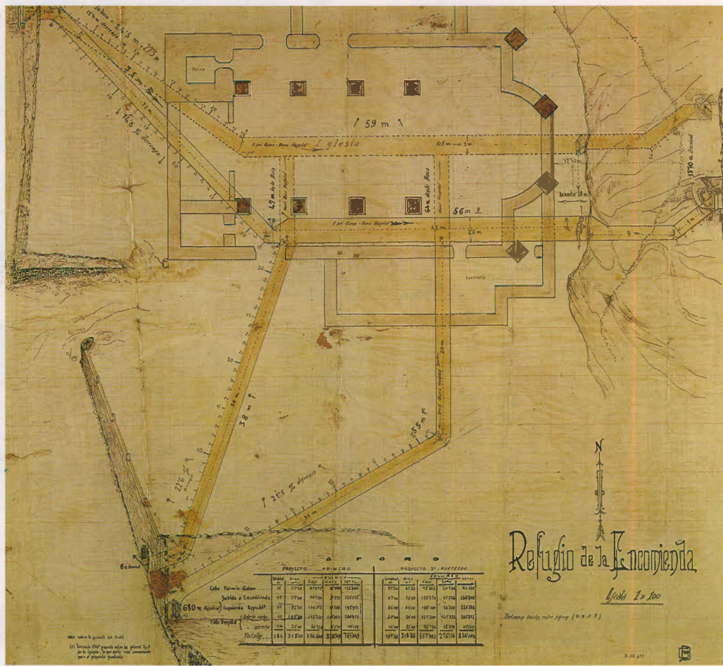
Refugio de «La Encomienda», construido en el año 1937.
